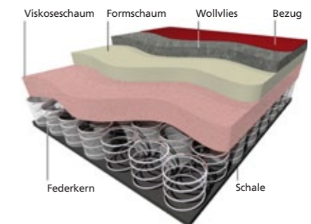
Komfortsitz, optional: Atmungsaktives, viskoelastisches Material nimmt Körpergewicht und -kontur vollständig auf. Die entstehende Druckentlastung schont Bänder, Sitzbeinhöcker, Muskulatur und Nerven. Im Gegensatz zu herkömmlichen Schaumstoffen fördert die kugelförmige, offene Zellstruktur der Viskose die gleichmäßige Verteilung des Körpergewichtes, vermeidet Druckstellen und fördert die Durchblutung. Die anatomisch exakte Unterstützung verhindert Fehlhaltungen.
